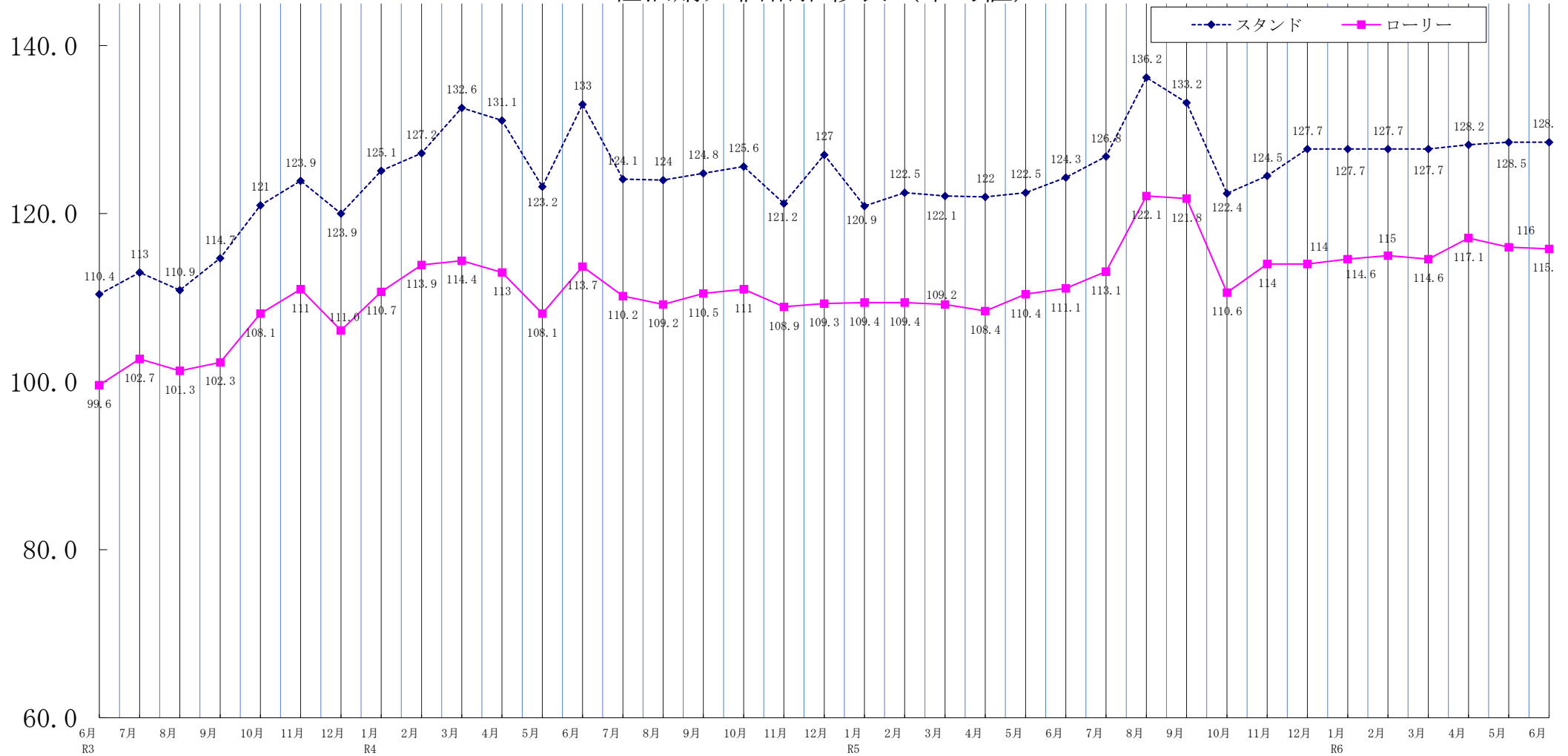
軽油購入価格推移表（平均値）
